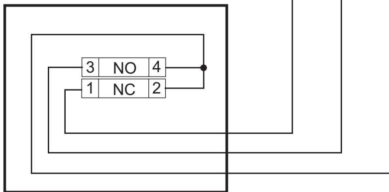
SFC VSS Vridströmställare (0-1-2)
